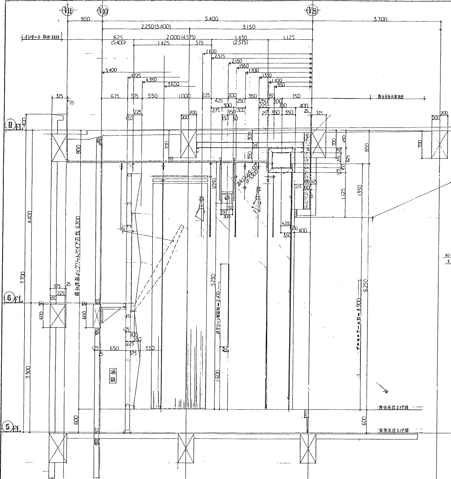
舞台吊物装置断面図
