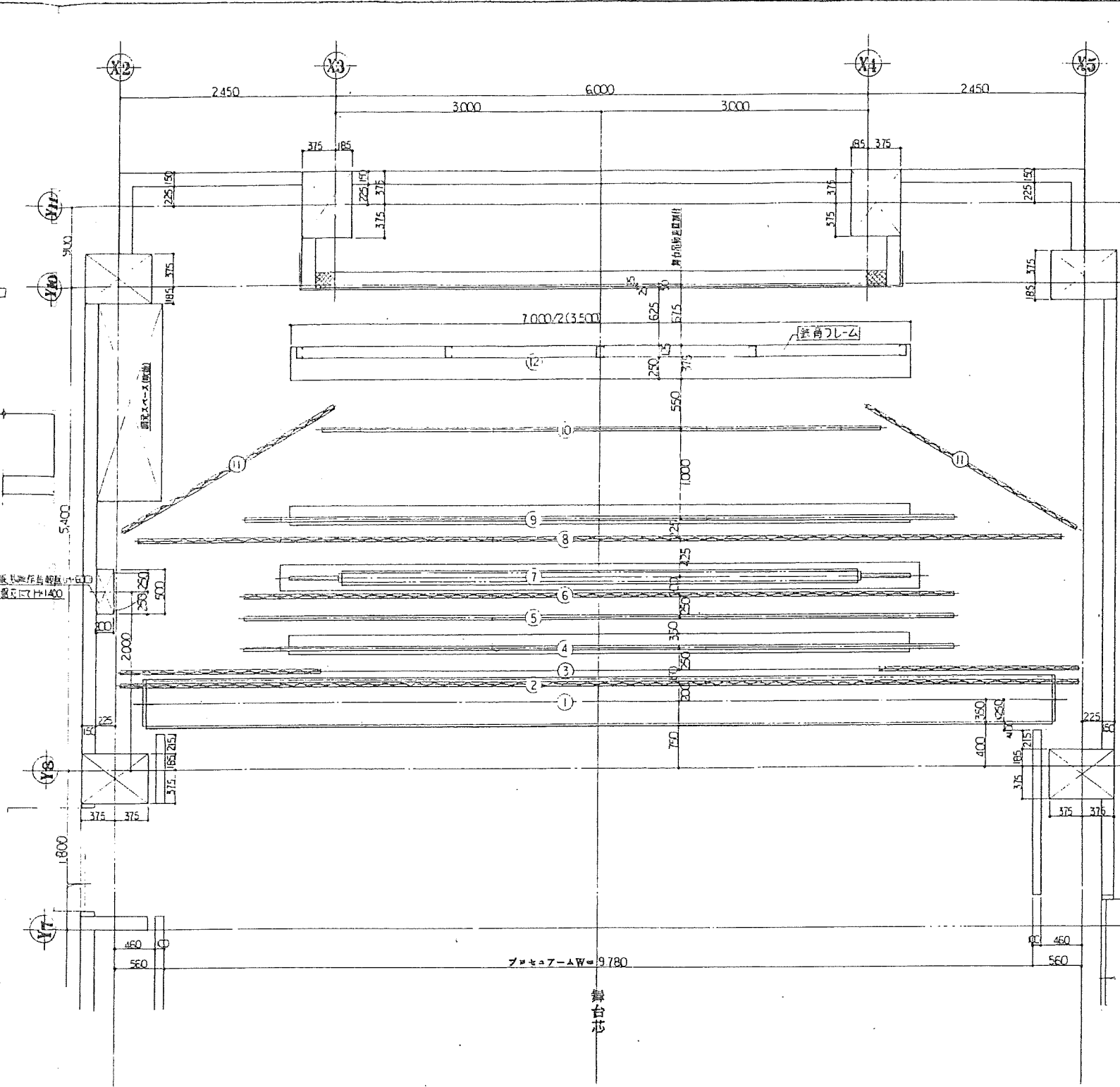
舞台吊物装置平面図
